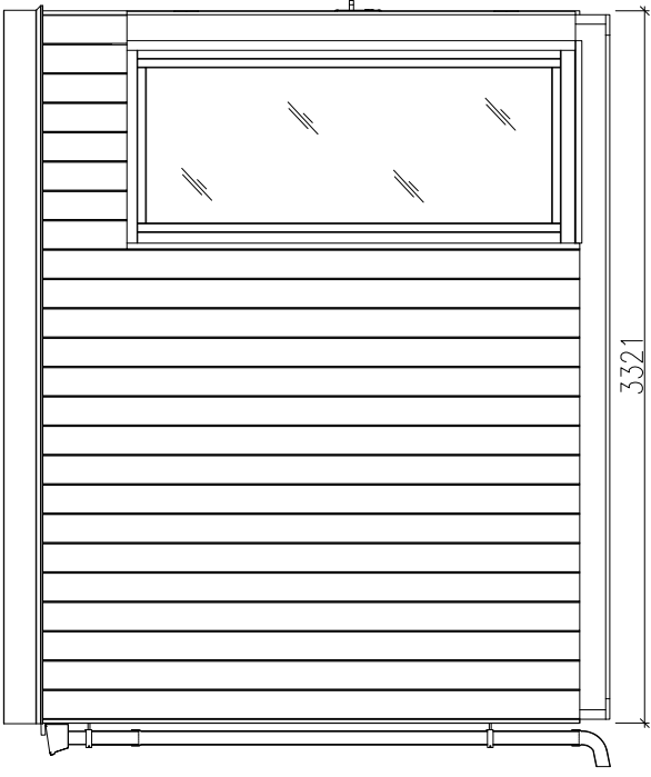
Left 1:50
